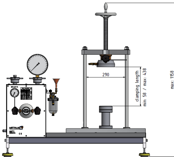
Oberholm-Option Vorderansicht Head Beam option front view
